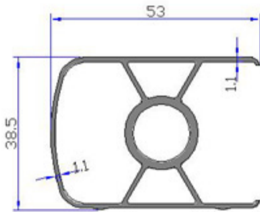
6210 - 0,825 kg/m
