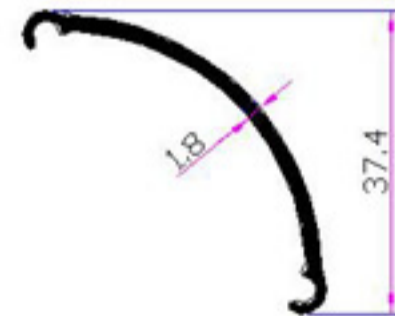
5296 - 0.290 kg/m
