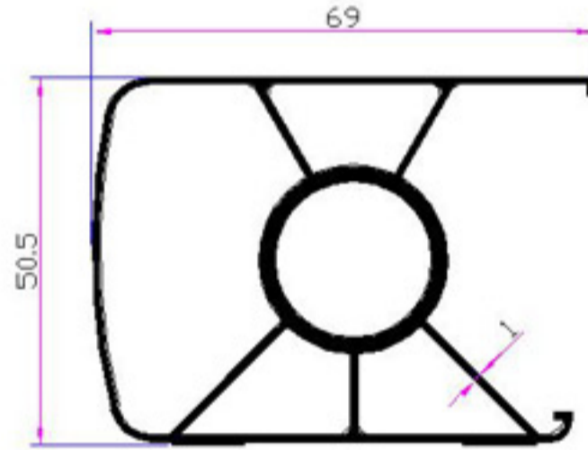
5187 - 1.153 kg/m
