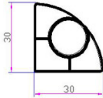
5215 - 0.500 kg/m
