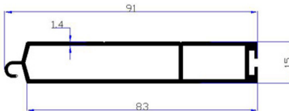
4268 - 0,795 kg/m
