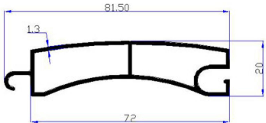
3957 - 0,750 kg/m
