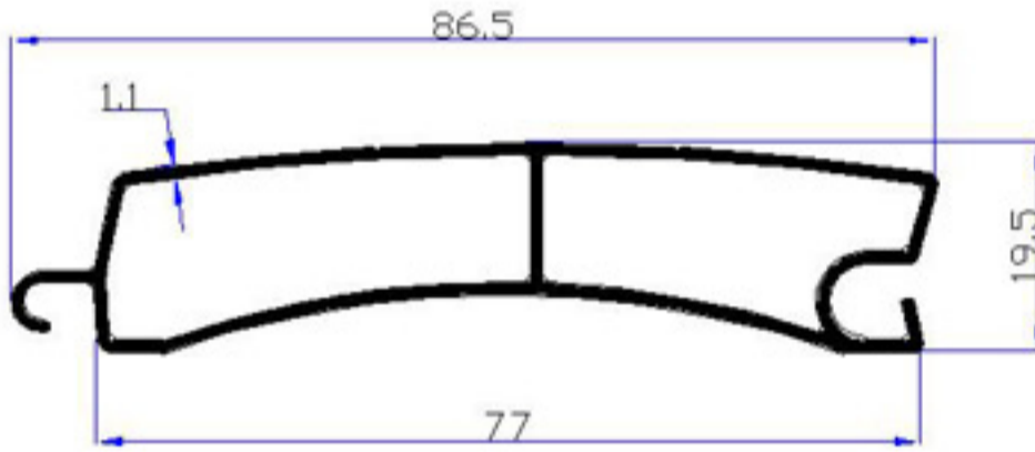
4531 - 0,655 kg/m
