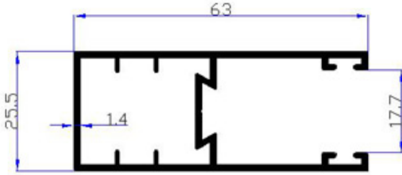
5670 - 0,770 kg/m
