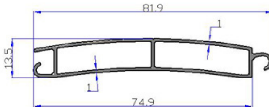
7293 - 0,527 kg/m
