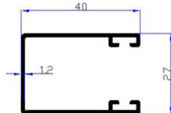
4313 - 0,430 kg/m
