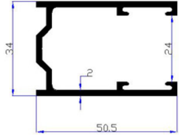
7006 - 0,820 kg/m
