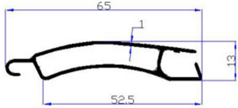
3733 - 0,400 kg/m
