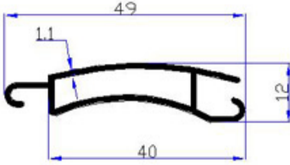
3597 - 0,320 kg/m
