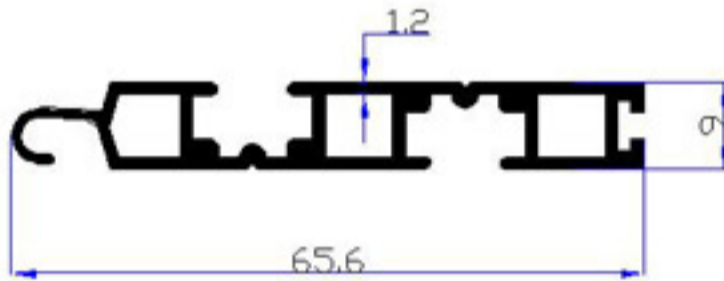
4549 - 0,588 kg/m
