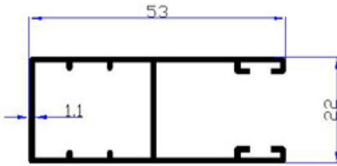
4273 - 0,502 kg/m
