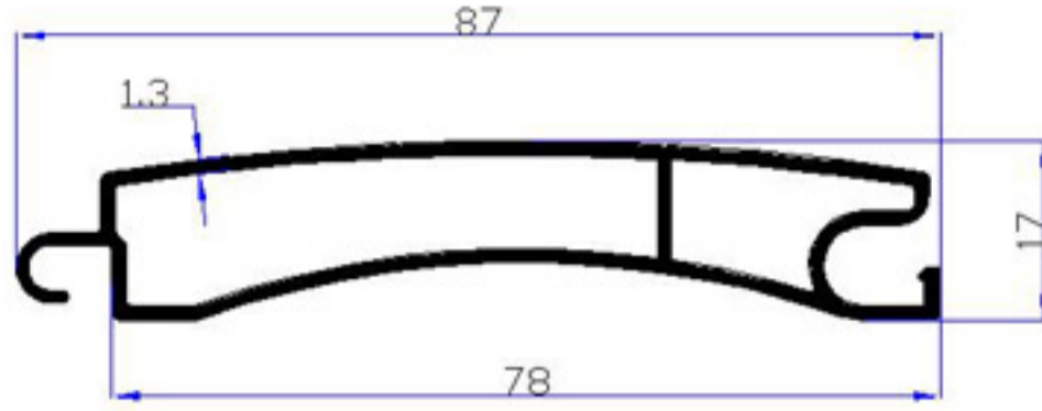
4317 - 0,756 kg/m
