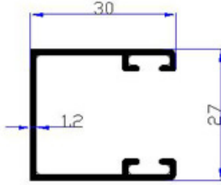
4495 - 0,340 kg/m
