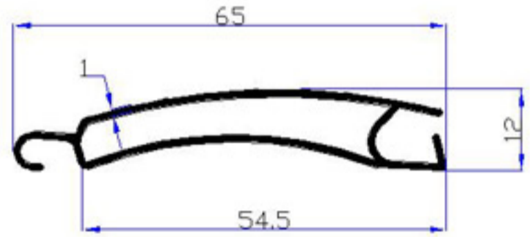
4548 - 0,417 kg/m
