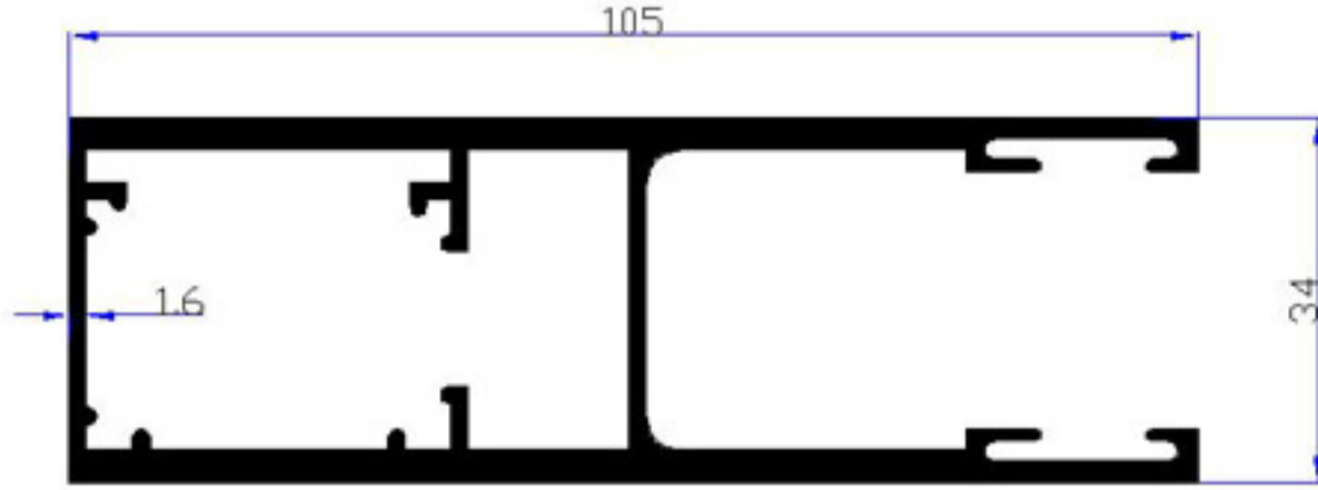
4314 - 2,080 kg/m
