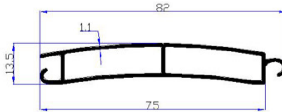
5635 - 0,580 kg/m
