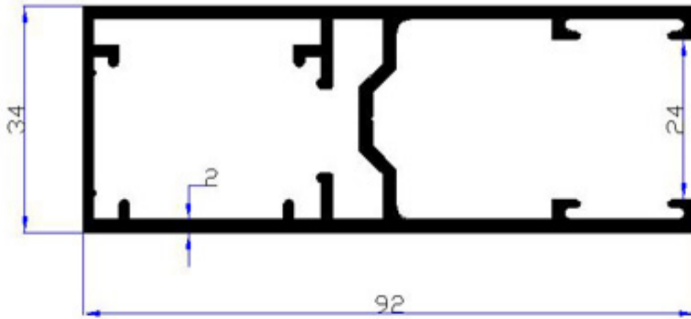
7007 - 1,550 kg/m
