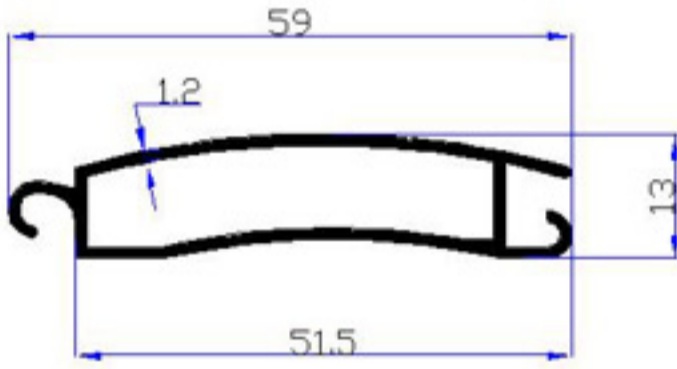
3955 - 0,450 kg/m
