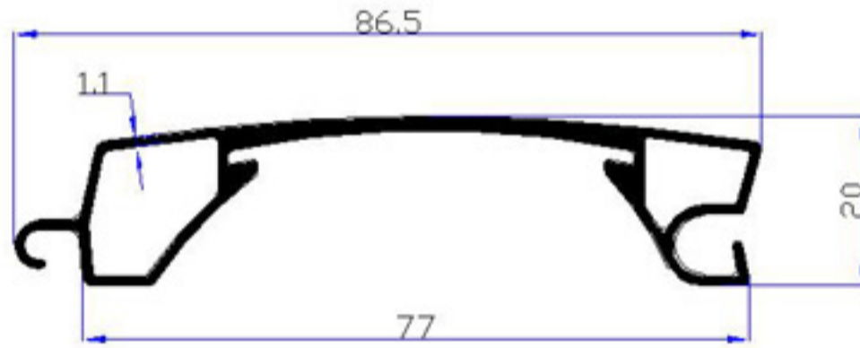
4532 - 0,760 kg/m
