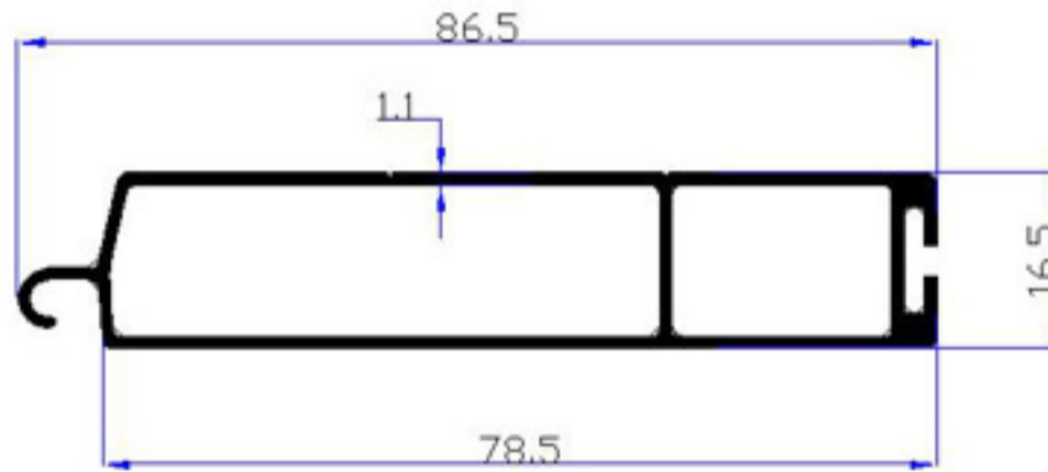
4533 - 0,690 kg/m
