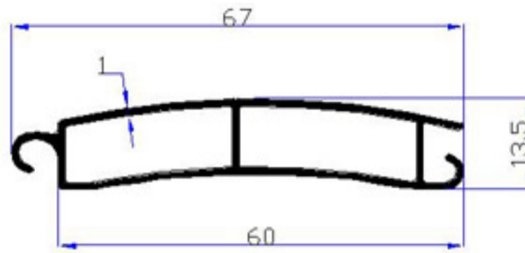
5634 - 0,450 kg/m
