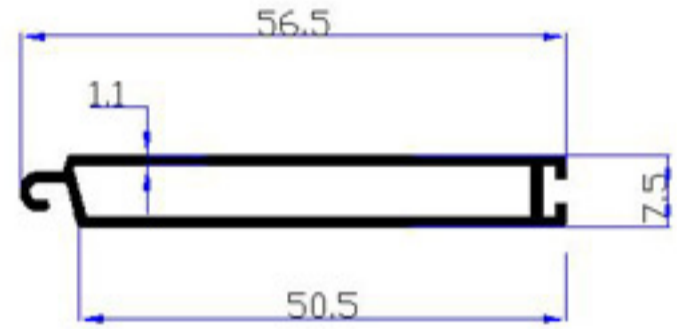
4274 - 0,375 kg/m
