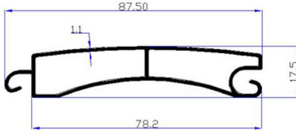
6655 - 0,685 kg/m
