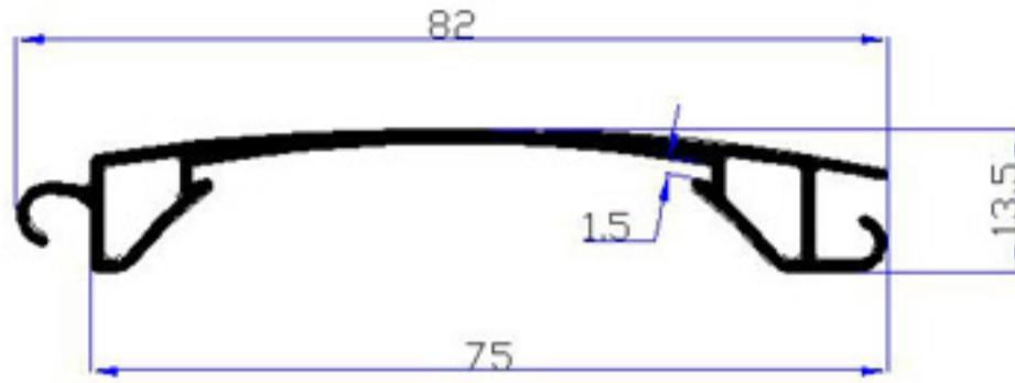
5633 - 0,545 kg/m
