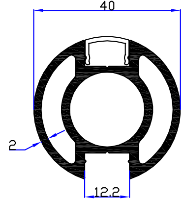
5231 - 1,135 kg/m
