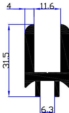
6710 - 0,730 kg/m
