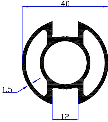
6541 - 0,933 kg/m
