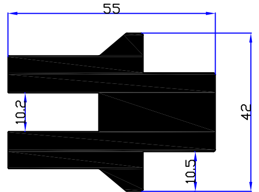
5392 - 3,600 kg/m
