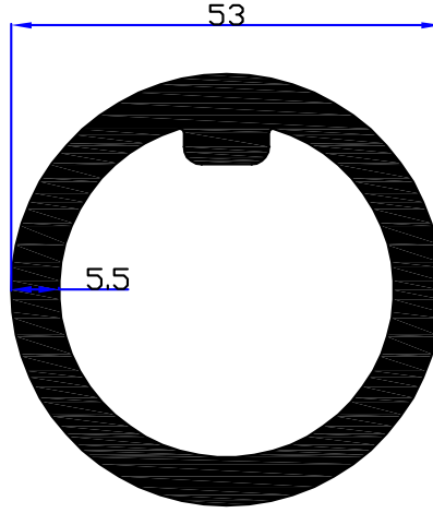
6652 - 2,495 kg/m
