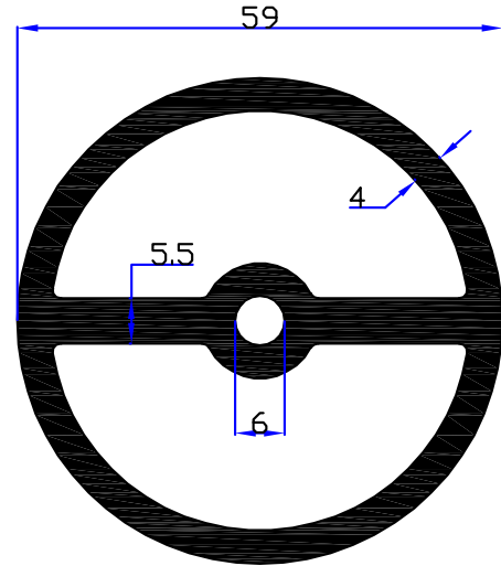
6707 - 2,770 kg/m
