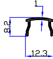
6542 - 0,070 kg/m
