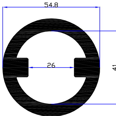
5394 - 3,220 kg/m
