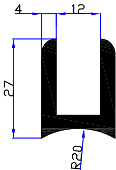
6709 - 0,666 kg/m
