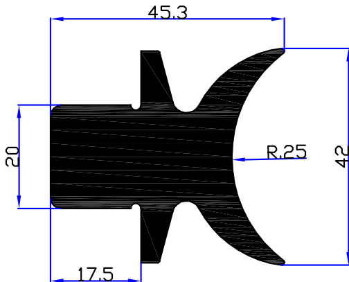
6712 - 2,580 kg/m
