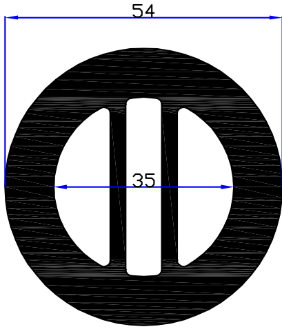
6708 - 4,150 kg/m
