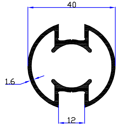
6699 - 0,770 kg/m
