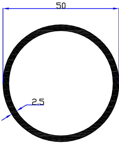
4619 - 1,090 kg/m
