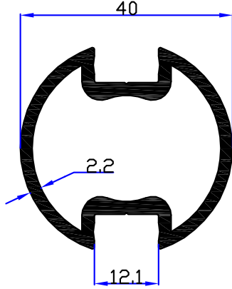
4624 - 0,900 kg/m
