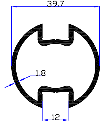
6540 - 0,737 kg/m
