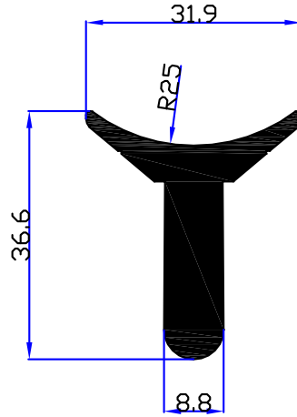
6654 - 0,970 kg/m
