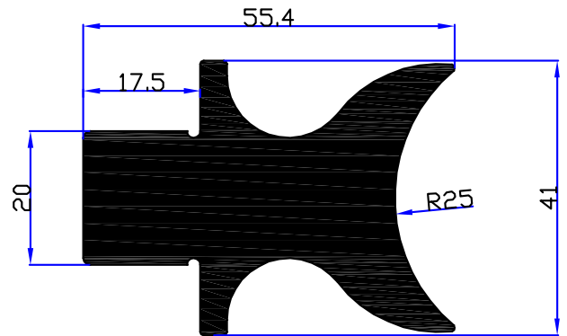
6713 - 3,380 kg/m
